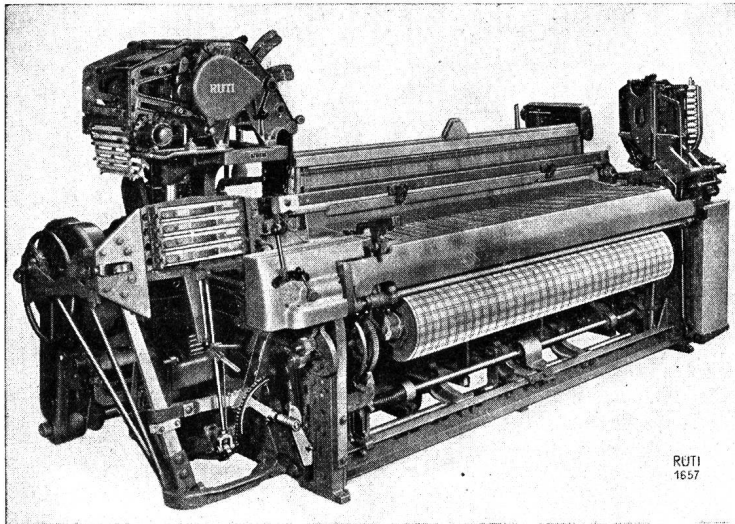
4-schütziger Buntautomat BANW/4 mit RH-Schaffmaschine
