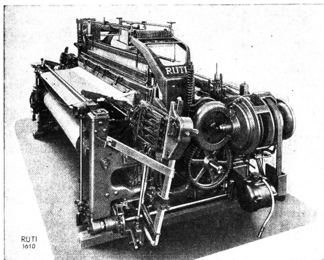
Rüti Pick-Pick Woll-Lancierstuhl TRU/7 mit leichtem Oberbau
