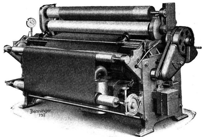
Benninger Gewebe-Absaugmaschine SRM
