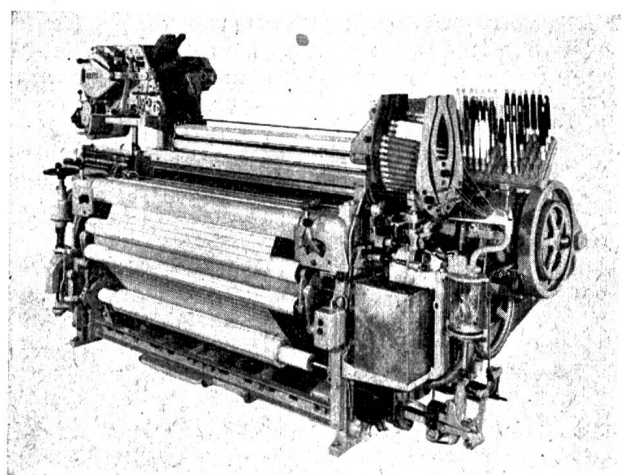
Rüti-Spulenwechsel-Webautomat SINZAW/4
