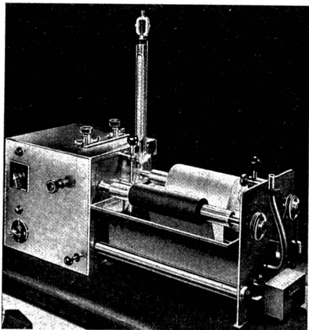
Automatischer Labor-Jigger
