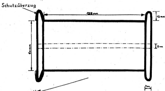
KONISCHE SCHEIBENSPULE FUER KOPFABZUG Typ 2
