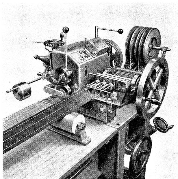
Der stationäre Bindemechanismus der Blattbindemaschine Typ BBiE. Das werdende Webeblatt wird von rechts nach links gezogen.
