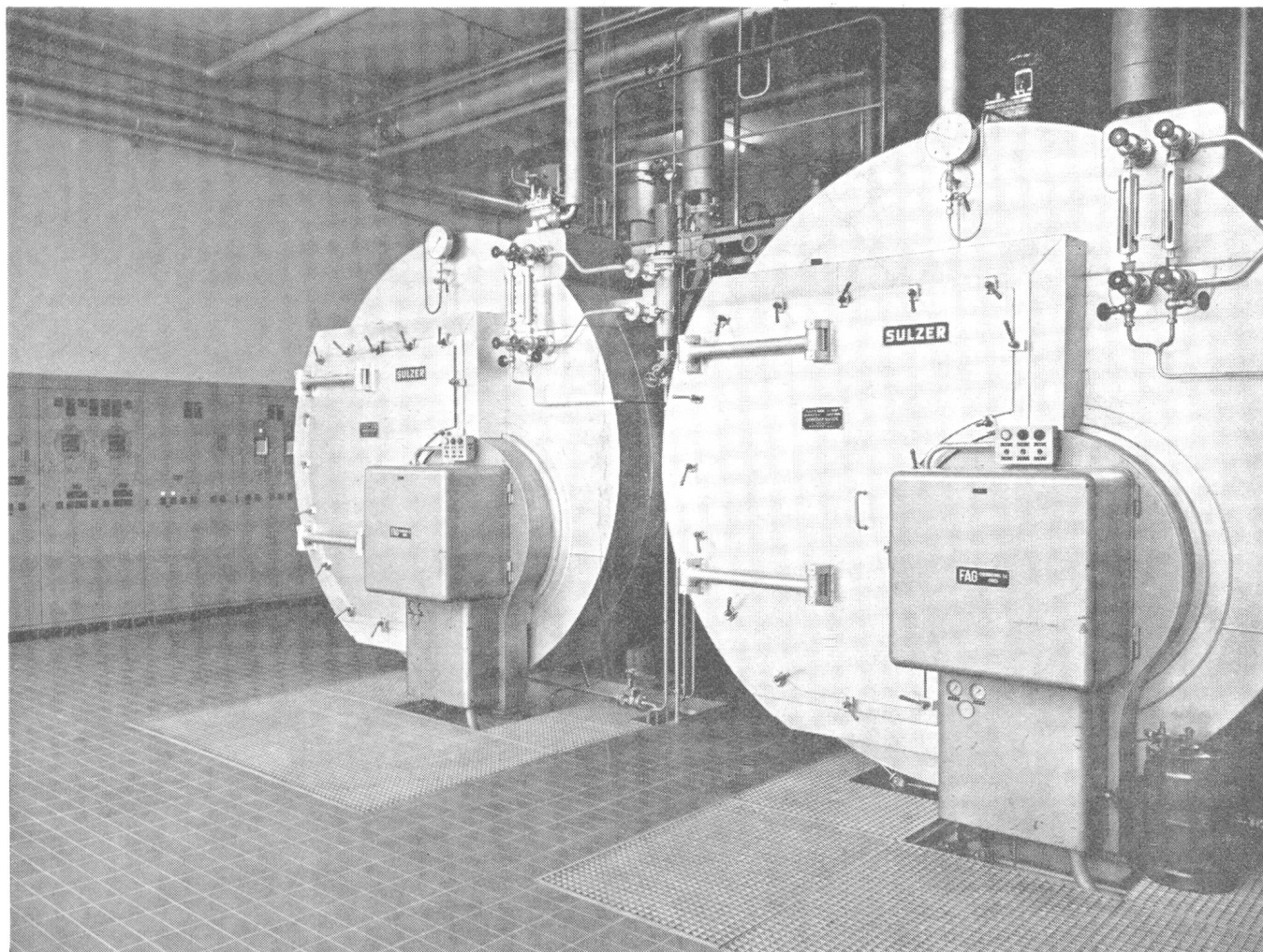
Frontansicht von zwei ölgefeuerten Dreizugkesseln in kompakter Bauart in einer Brauerei. Sämtliche der Inbetriebsetzung, Steuerung und Überwachung der Kessel dienenden Meßinstrumente und Schaltapparate sind auf einer zentralen, an der Kesselhauswand aufgestellten Instrumententafel zusammengefaßt.
