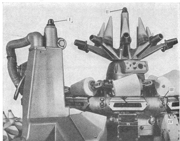
Oberteil des Schweißer-Rundautomaten mit den Signallampen I-IV. Oberhalb des Spltisches erkennt man das Steuergerät der elektronischen Fadenreiniger sowie die Halterung mit den Aufsteckzapfen für Vollkone und den Reserve-Konehüllen.
