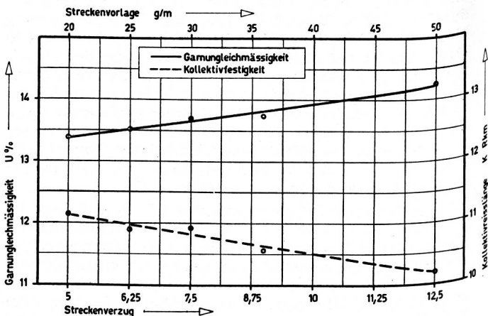
Abb. 4 Garnungleichmäßigkeit und Kollektivfestigkeit in Abhängigkeit der Fasermasse
