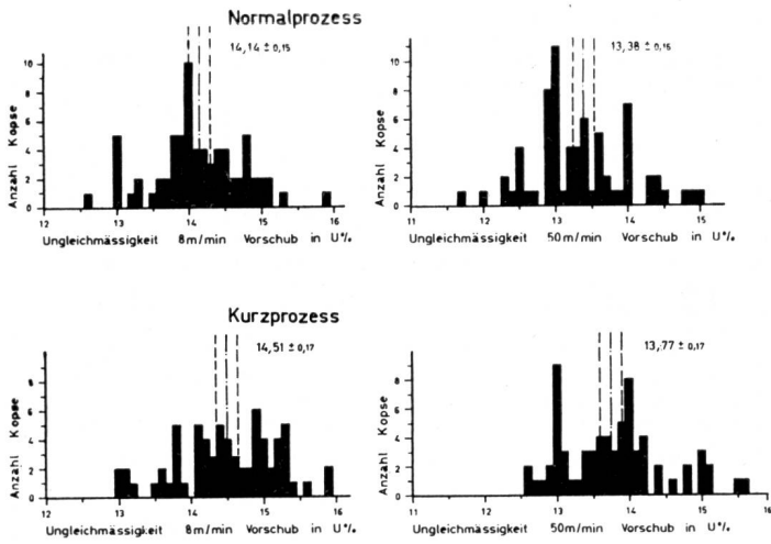
Abb. 9 Garnungleichmässigkeit
