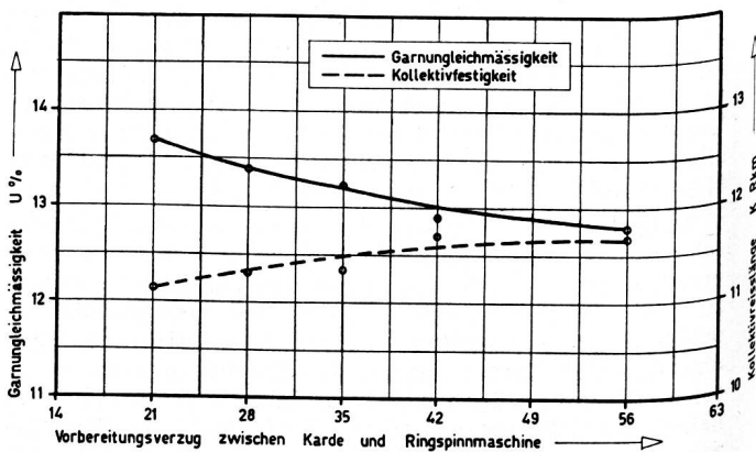
Abb. 3 Garnungleichmäßigkeit und Kollektivfestigkeit in Abhängigkeit des Vorbereitungsverzuges
