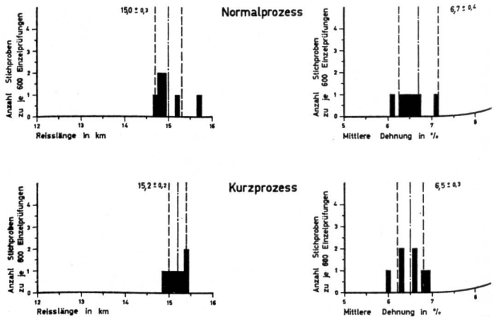
Abb. 13 Einzelfadenfestigkeit und Dehnung, Dynamometer «Uster»
