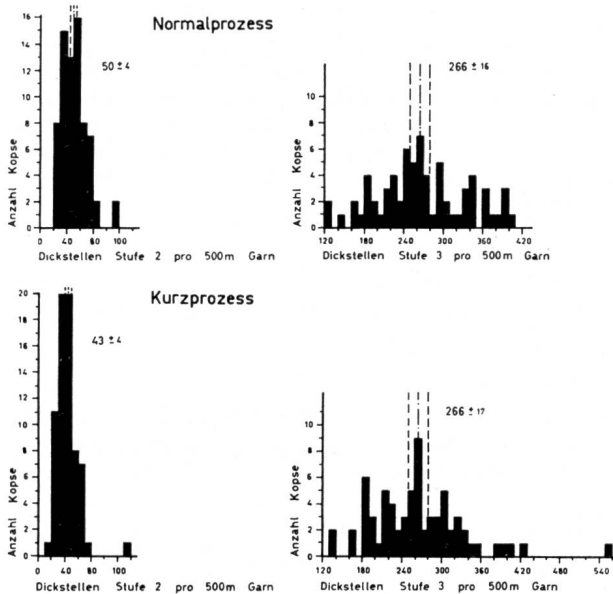
Abb. 11 Dickstellen IPI
