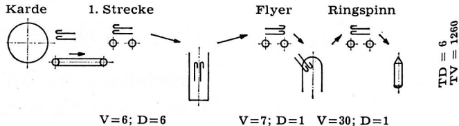
Abb. 1 Vergleich konventioneller Spinnprozeß zu abgekürztem Spinnprozeß, Lage der Fasern mit Schlepphaken, Dublierung und Gesamtverzug
