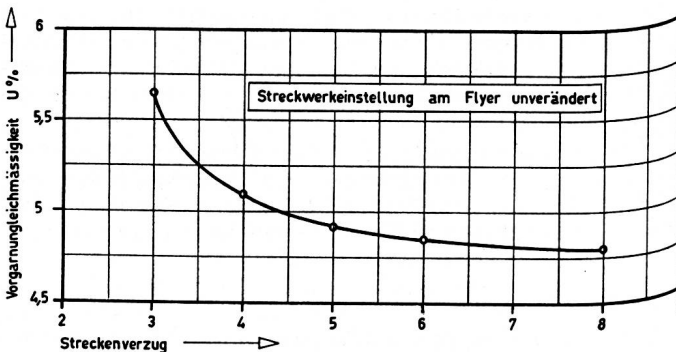
Abb. 2 Vorgarnungleichmäßigkeit in Abhängigkeit des Streckenverzuges
