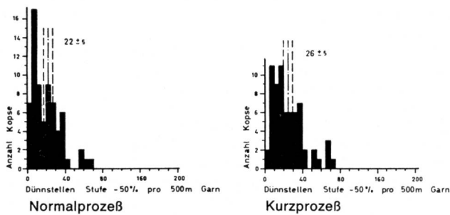
Abb. 10 Dünnstellen IPI
