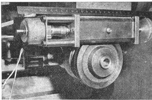
Digitalmotor mit elastischer Kupplung treibt über ein Getriebe 100 : 1 die Vorschubspindel an
