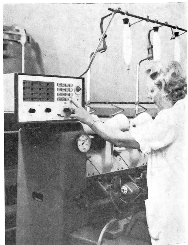
CLASSIMAT-Garnfehlerklassieranlage auf Prüfpulmaschine
