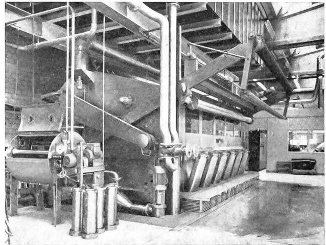
Moderne Stückfärbearlage für 5 m breite Teppichbahnen (Elektronisch gesteuert)
