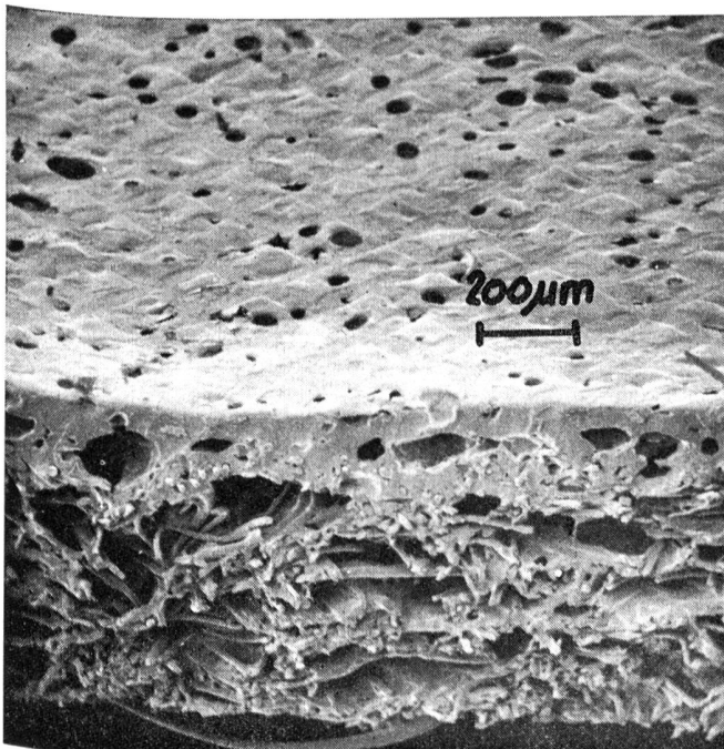
Abbildung 12 Synthese-Leder-Anschnitt
