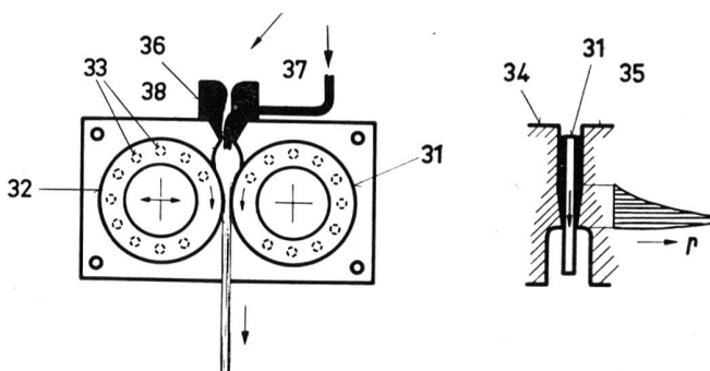
Abbildung 12 Imprägnierkopf (schematisch)
