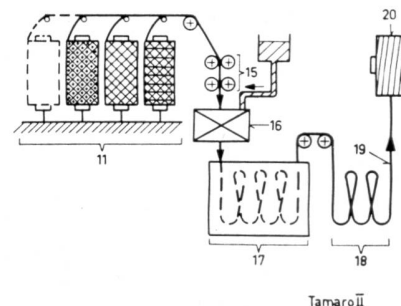
Abbildung 21 Paset-Garn (geklebt)
