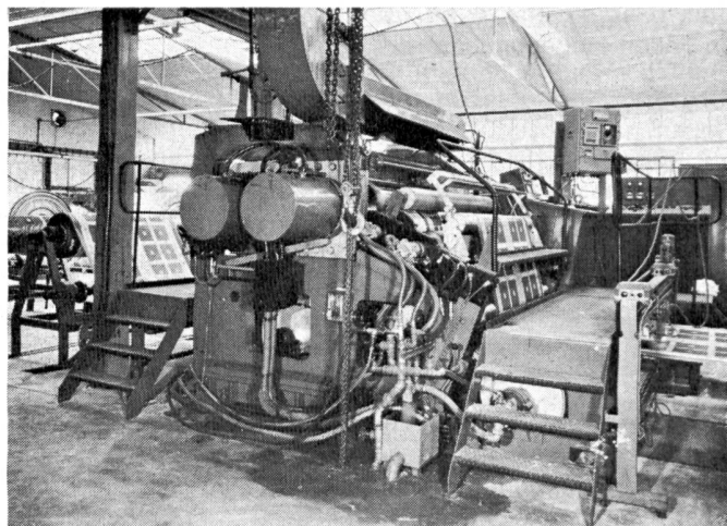
Abbildung 5 Walzenschmelzmaschine mit 1600 mm Arbeitsbreite (Zimmer Plastic GmbH, Offenbach).
