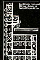
Kombinierter Horizontal- Länder 4-bahig mit Vertikal-Etagenländer
