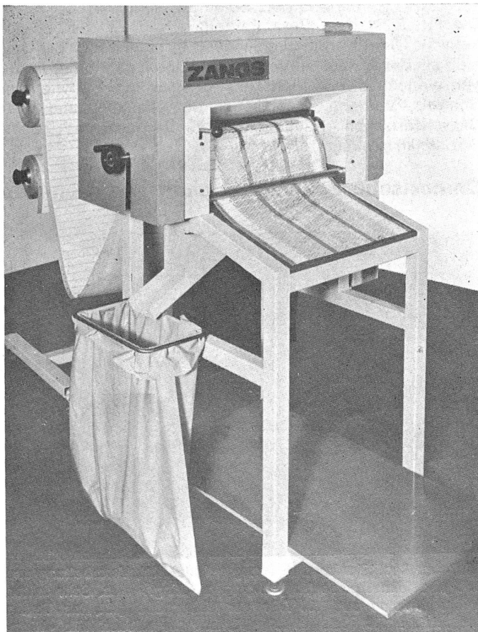
Kartenschnellstanze Patropunch® 528 innerhalb des Zangs-Patrocard-Systems® 525, einem rechnergesteuerten Verarbeitungssystems der Jacquard-Ateliertechnik, mit Abrolleinrichtung 527 für gerolltes Kartenpapier.
