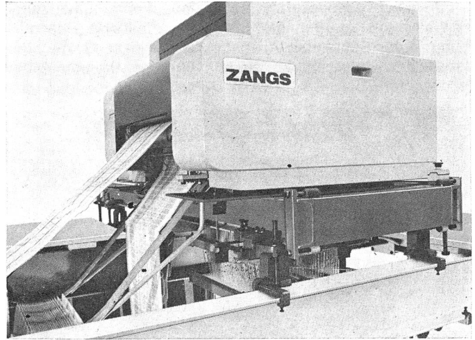
Zangs-Jacquardmaschine 356 Doppelhub-Ganzoffenfach mit Schrägfach, 1344 Platinen.
