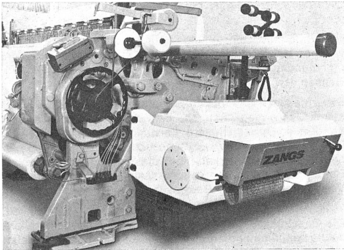
Zangs-Gegenzug-Rotationsschiffmaschine 440 für vielschäftiges Weben bei hohen Touren und grosser Blattbreite.
