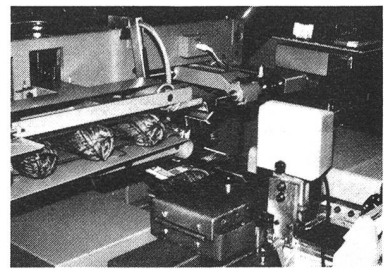
Banderolieren der Knäuel unmittelbar nach dem Wickeln
