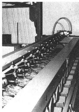
Blick in die Wickelmaschine
