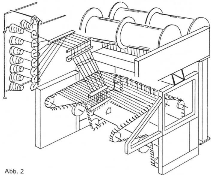
Anwendungsgebiet der hochfesten Nylsuisse- und Tersuisse-Garne: Beschichtungs- und Gummierungsgewebe, für Lastwagenplanen, Traglufthallen und ähnliches.
