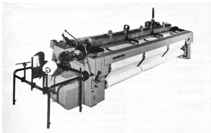
Sulzer Rütli Projektilwebmaschine des Typs PS 4000 ES E6 in niedriger Bauart mit einer max. Arbeitsbreite von 4000 mm, ausgerüstet mit Exzentermaschine
