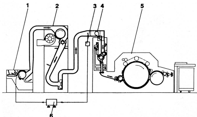
Bild 2 Schnittzeichnung: Elektronische Steuerung Contifeed CF 1. Reiniger RSK 2. Kondensator LVSB mit Ventilator TVF 425 3. Druckaufnehmer 4. Flockenspeiser Exactafeed® FBK 533 5. Hochleistungskarde Exactacard® DK 715 6. Regler mit Einstellung für Grunddrehzahl und Druck-Sollwert
