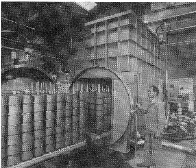
Die mikroprozessorgesteuerte Horizontalfärbemaschine Ecobox der französischen Firma Barriquand in Roanne zeichnet sich durch ihren platzsparenden Aufbau und durch die gleichbleibend hohe Qualität des reproduzierbaren Färbeergebnisses aus.
