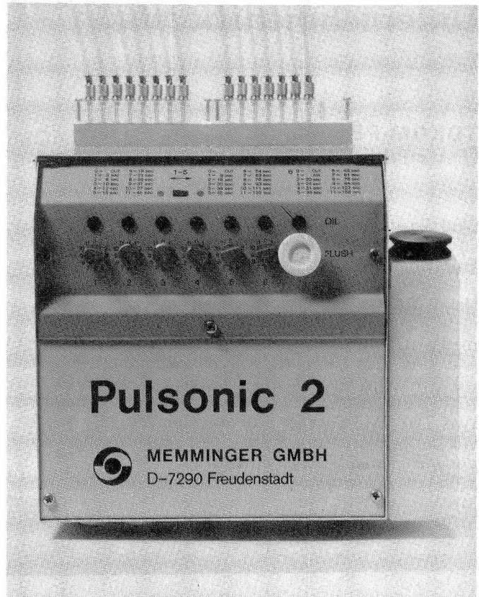
Pulsonic-2 «Maxi» für 1–15 Ölstellen mit 3,5 l Ölbehälter und elektronischer Ölflussüberwachung mit Maschinenstopp, wenn in einem der Druckschläuche kein Öl fliesst. Visuelle Ölflussüberwachung ohne Maschinenstopp auf Kundenwunsch. Bei beiden Überwachungsarten Maschinenstopp bei Erreichen des Min.-Ölstandes. Einstellbare Schmierintervalle für Gruppen von je 3 Pumpen. Sonderzubehör: Nadelungenschmierung mit 1 oder 2 Sprühdüsen, die für eine einwandfreie Verneblung sehr geringe Mengen Luft und Öl benötigen.
