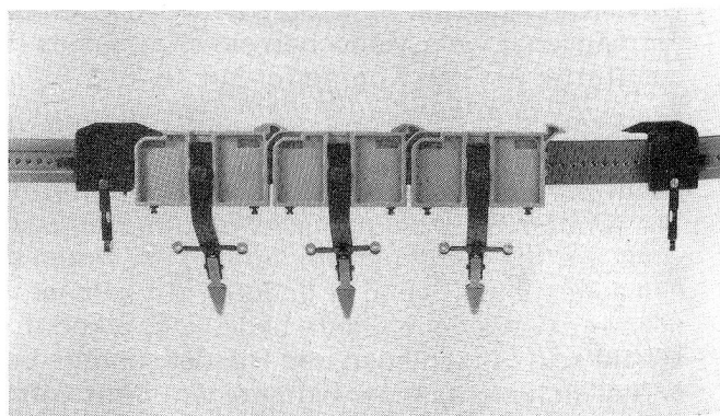
Die Abbildung zeigt den Anwendungsfall als Mehrfachkasten; drei Fadenführerkästen arbeiten auf einer Spur zusammen.
