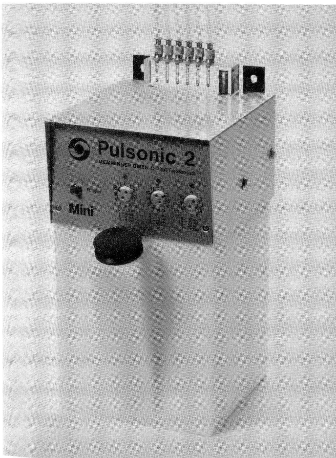
Pulsonic-2 «Mini» für 1–6 Ölstellen mit 2 l Ölbehälter, visueller Ölflussüberwachung und automatischem Maschinenstopp bei Erreichen des Min.-Ölstandes. Einstellbare Schmierintervalle für Gruppen von je zwei Pumpen.
