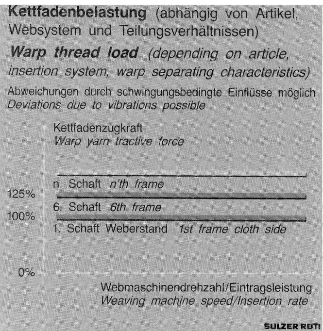
Abb. 7 Kettfadenbelastung
