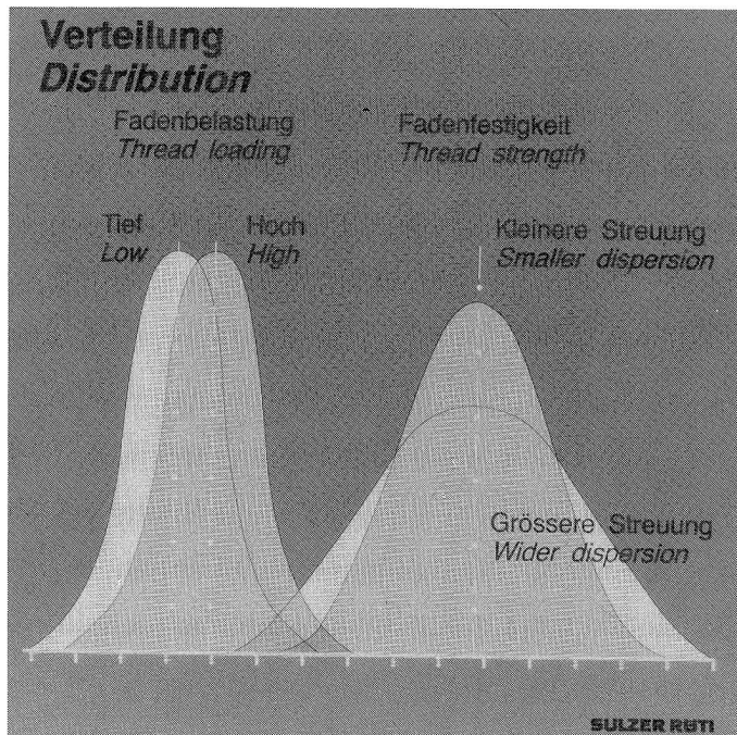
Abb. 8 Verteilung
