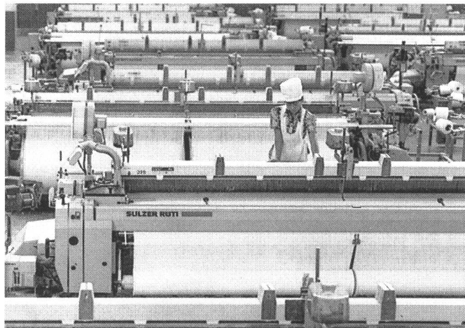
Webmaschinenanlage der Handan Cotton Mill mit 50 Sulzer Rüti Projektilewebmaschinen, auf denen das Unternehmen mehrbahnig hochwertigen Popeline herstellt. Das vollstufige Unternehmen beschäftigt 8000 Mitarbeiter und gehört mit 100 000 Spindeln und 2600 Webmaschinen zu den grössten Textilunternehmen in China. Das Produktprogramm reicht vom leichten und mittelschweren Baumwollkörper bis zum feinen Popeline und Inlett. Mehr als 90 % der Gewebe werden exportiert. Bild: Sulzer Rüti
