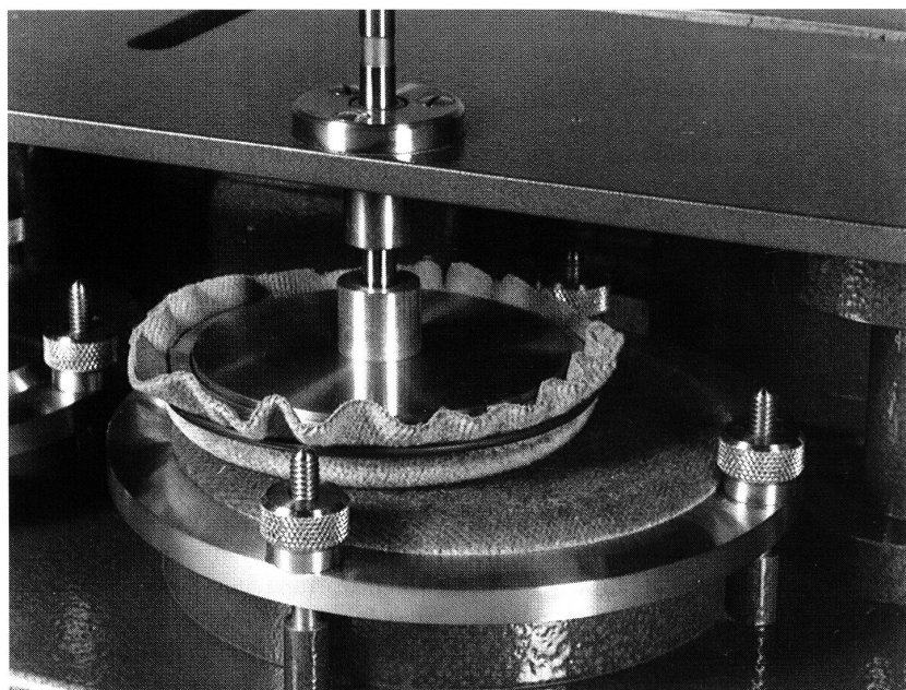
Der Martindale Scheuertester von James H. Heal & Co. Ltd.
