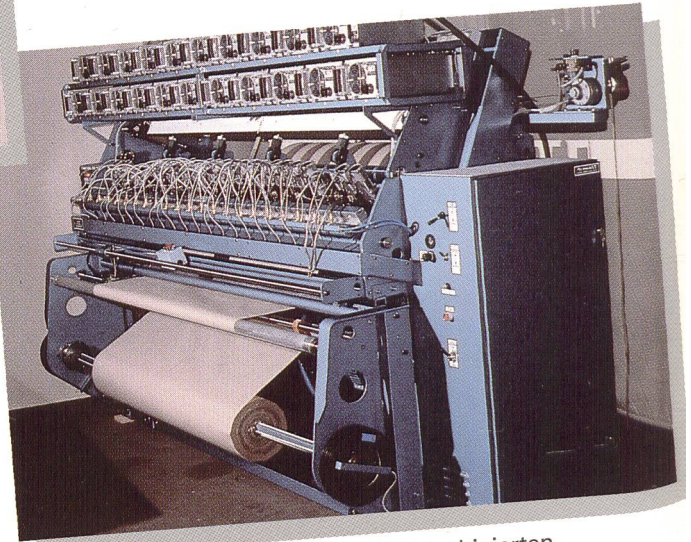
Schneidmaschine Type TF.BMT für kombinierten Ultraschallschweiss- und Kaltschnitt
