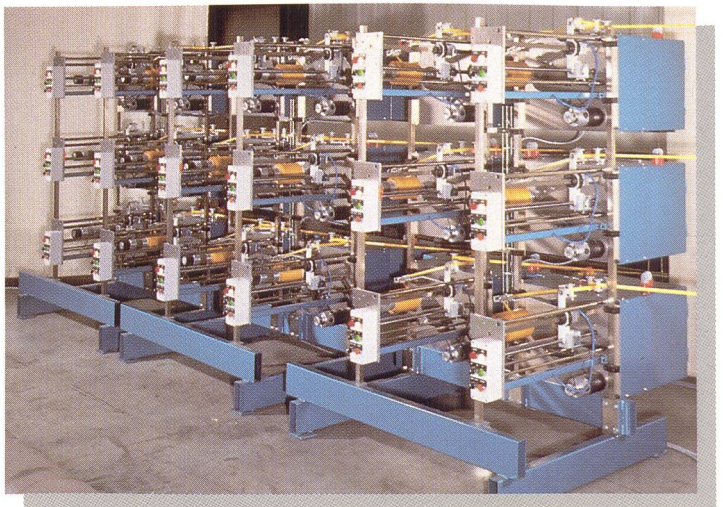
Kreuzwickelmaschine für Bänder
