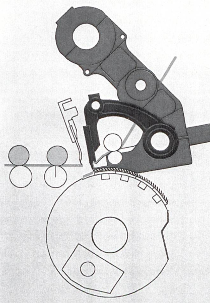
Kompaktzange
