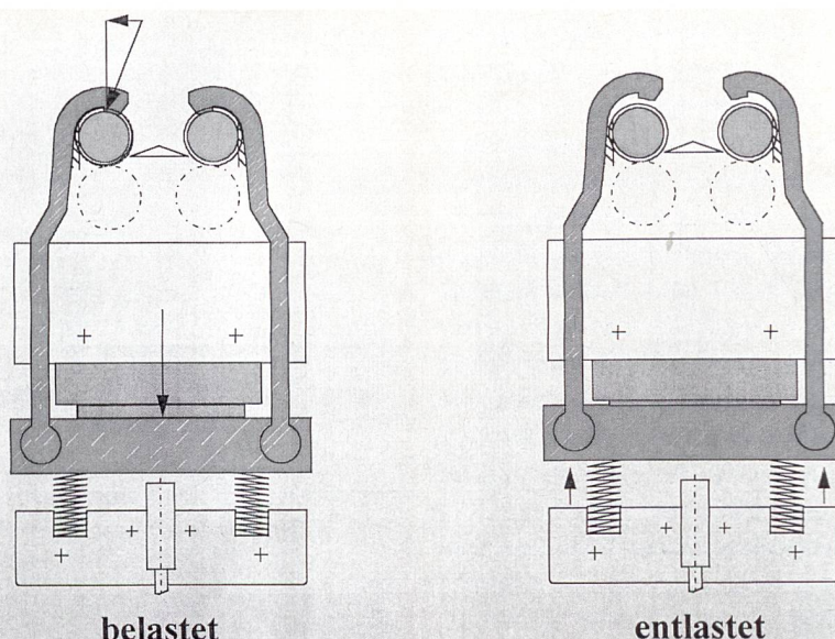
Pneumatisches AOW-Belastungssystem
