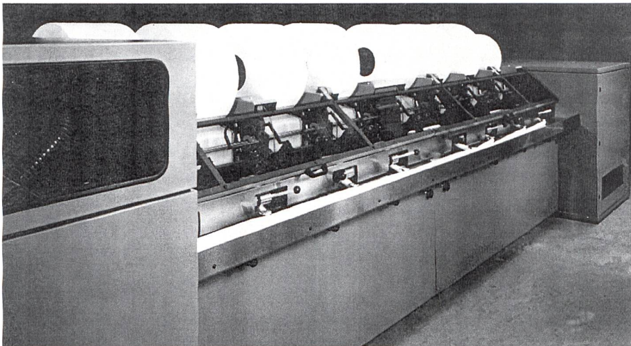
Kämmaschine Modell 1535
