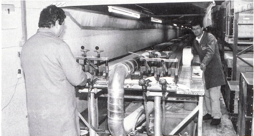
Bild 2: Gummierung
