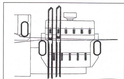
Abb. 2: Niederhaltevorrückung zur zusätzlichen Schonung der Kettfäden, Grob, Horgen (CH)
