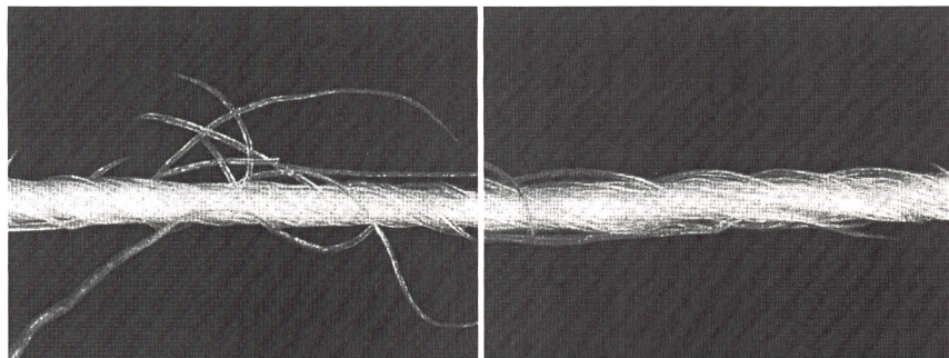
Vergleich der Garnstruktur, links konventionelles Ringgarn, rechts Solospun TM -Garn
