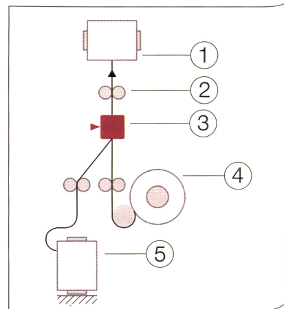
Abb. 5: Air-Covering-Verfahren
