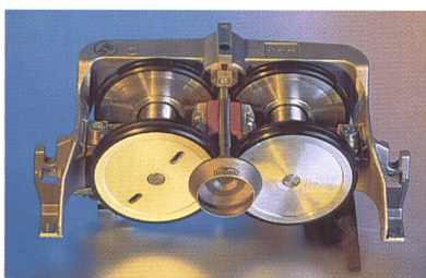
Rotormagnetlagerung «Twin-Coro»
