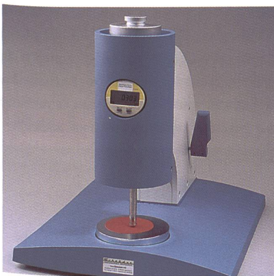
Dickenmessgerät der Firma Karl Schröder KG
