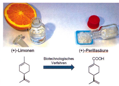
Abb. 3: Überführung von Limonen in Perillasäure
