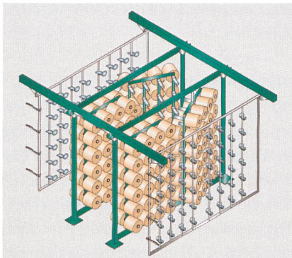
Abb. 3: Aufbauskinizze des Drebrahmengatters GD
