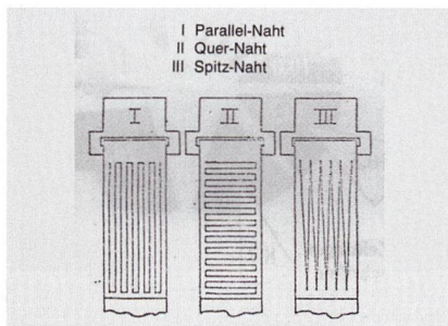
Abb. 8: Verschiedene Nahtformen
