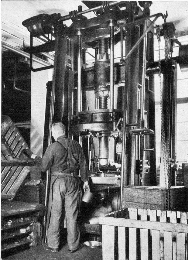
Räderziehpresse
