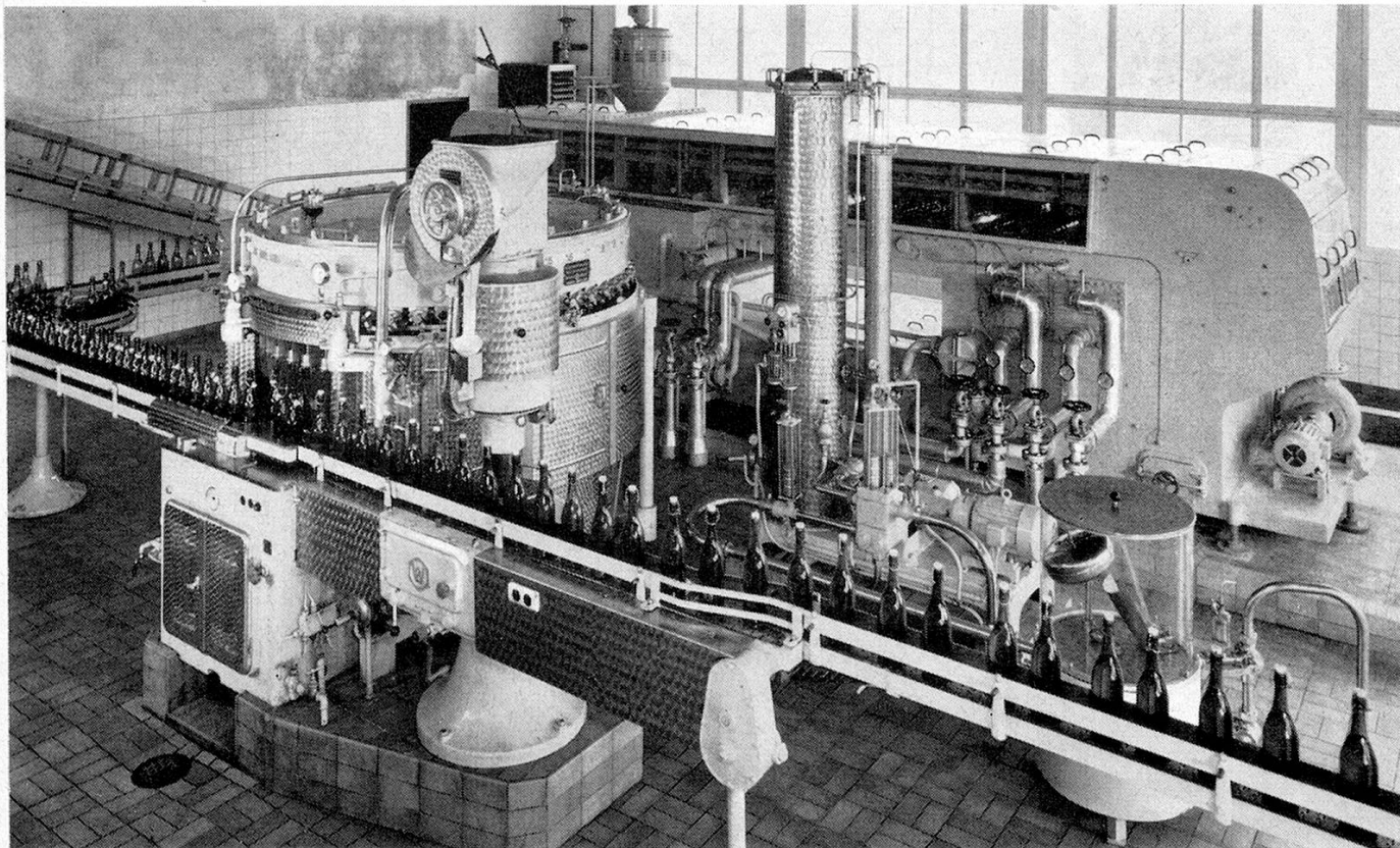
Blick in eine moderne Abfüllstation / Hintergrund: Flaschenwaschmaschine Mitte links: Flaschenfüller mit angebauter Kronenkork-Verschließanlage Harassen- und Flaschenförderband
