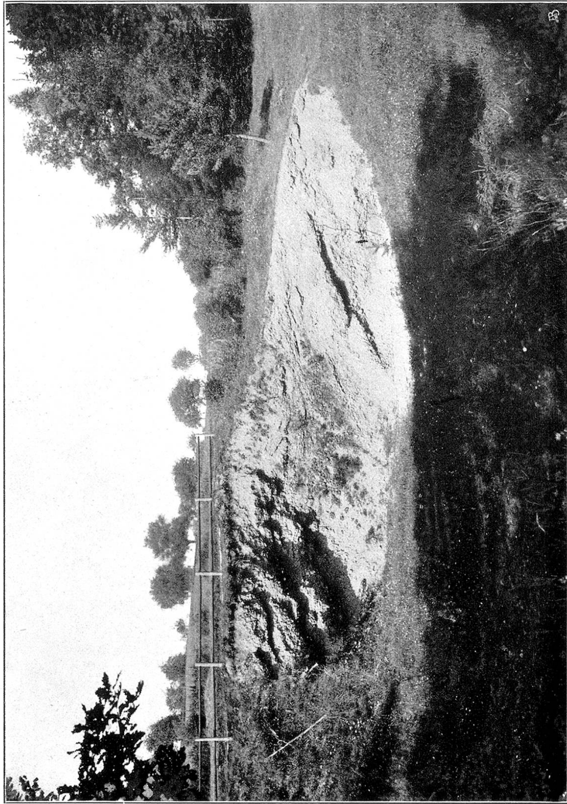
Aelterer Deckenschotter der Staats- und Gemeindekiesgrube W Reutenen. Ansicht S—N gegen die Straße. Uebergangsschicht abgetragen; nach NW und W fallende Nagelfluh. Aufnahme von Prof. Dr. Hefß.
