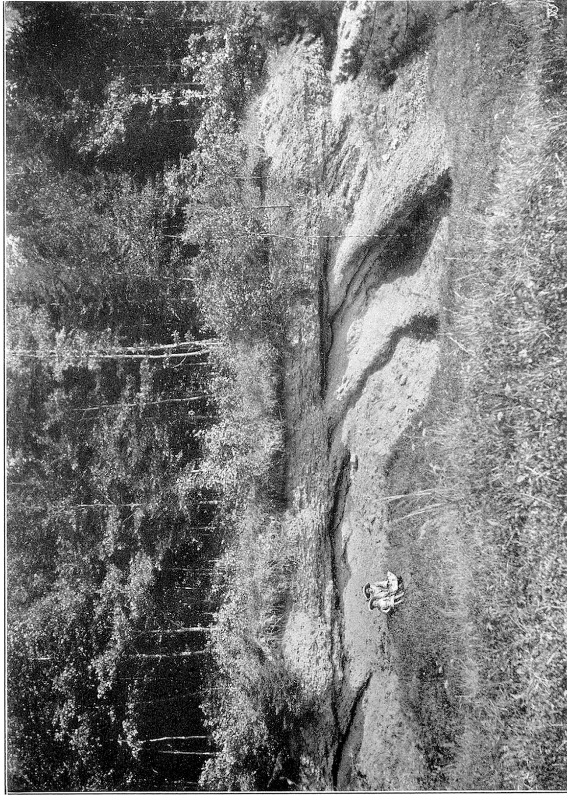
Älterer Deckenschotter der Staats- und Gemeindegroben W Reutenen.
