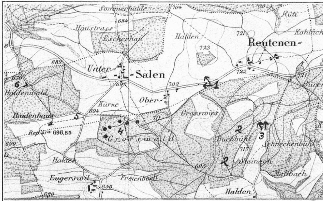
Fig. 1. Entblösungen (Zahlen und dicke Punkte im Großwald) des älteren Deckenschotters in Salen-Reutenen. Zahlen und Pfeile dem Text entsprechend. (Top. Atlas 1 : 25 000, Bl. 50).
