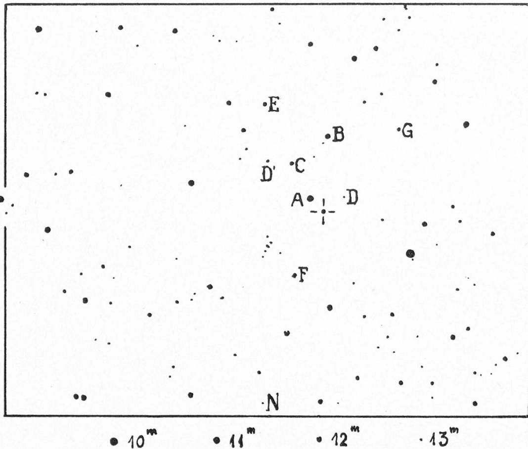
Fig. 1. Umgebung des «neuen Sterns» (+) im Sternbild des Schwans (Anblick im umkehrenden Fernrohr). Der Stern steht 15.8 Min. östlich, 1^{\circ}20' nördlich des Sterns \epsilon Cygni. Koordinaten: Rekt. = 20^{\text{h}}56^{\text{m}}13^{\text{s}} , Dekl. = +34^{\circ}44'.7 (1855.0). Maßstab der Karte: 1^{\circ} = 19.7 cm. Vergleichssterne: A 10^{\text{m}4} , B 11^{\text{m}7} , C 12^{\text{m}1} , D 13^{\text{m}3} , E 12^{\text{m}0} , F 12^{\text{m}1} , G 12^{\text{m}6} , D' 13^{\text{m}7}
