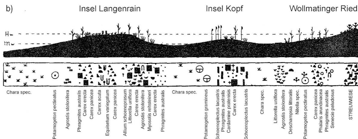
Abbildung 3: (a) Zwei Vegetationsprofile bei den Inseln im Wollmatinger Ried (Tafel XV aus Bauermann 1911a). Erläuterungen im Text; (b) Vegetationsprofil bei den beiden Inseln im Wollmatinger Ried (Profil 5 aus Bacmeister 1938), Pflanzennamen ergänzt. Erläuterungen im Text.
