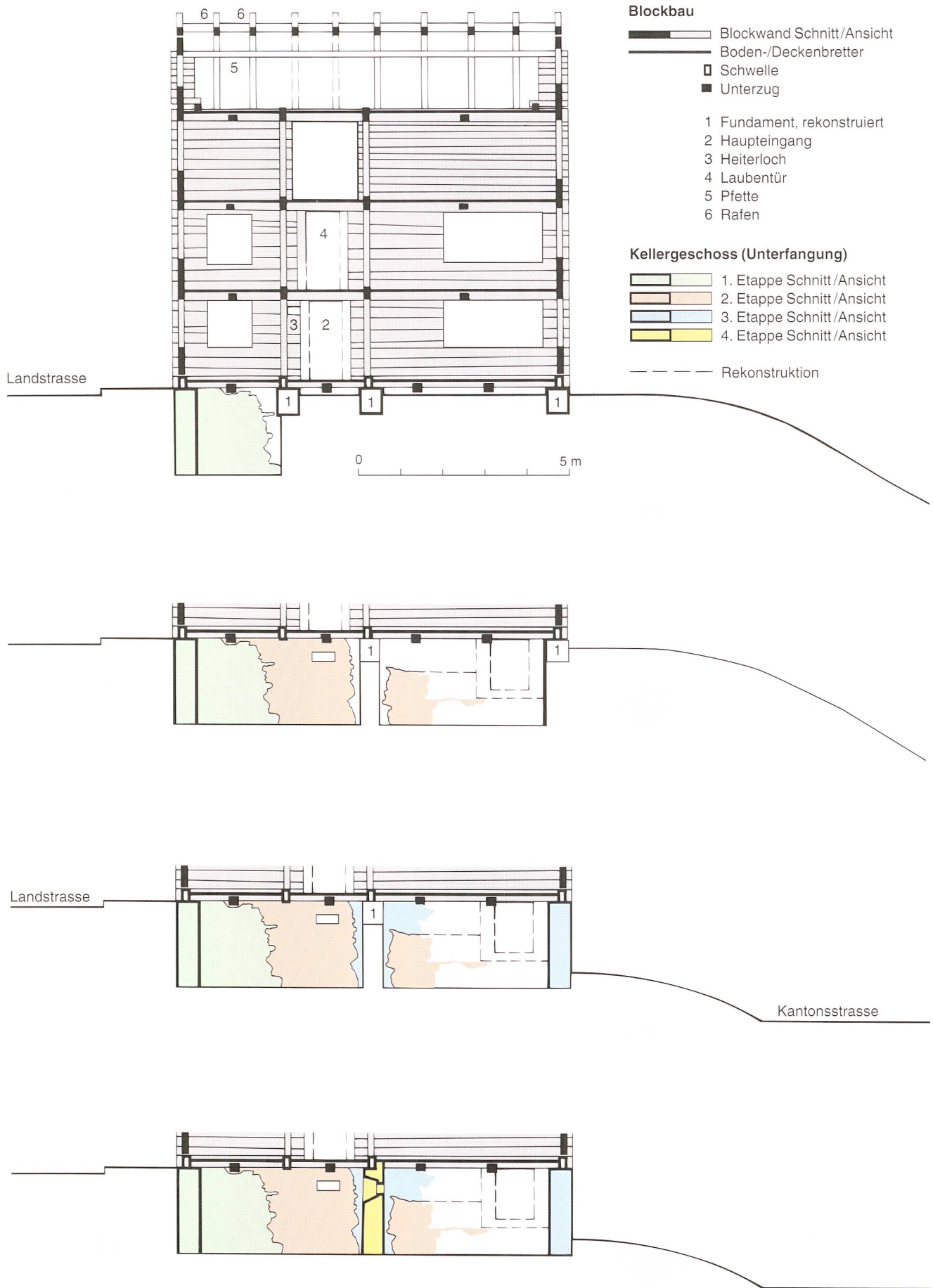
Abb. 6 Menzingen, «Kieferhaus». Schematischer Gebäudeschnitt Nord-Süd und Rekonstruktion der Unterfangungsetappen. Blick nach Osten.
