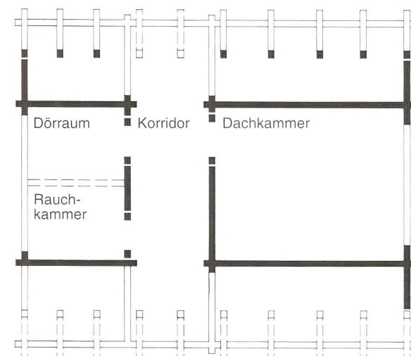
Dachgeschoss Blockbau
