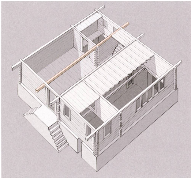
Abb. 3 Oberägeri, Haus Alosenstrasse 4. Perspektivische Rekonstruktion des unteren Wohngeschosses mit orange markiertem transversierendem Querbalken zur Stabilisierung des Blockgefüges.
