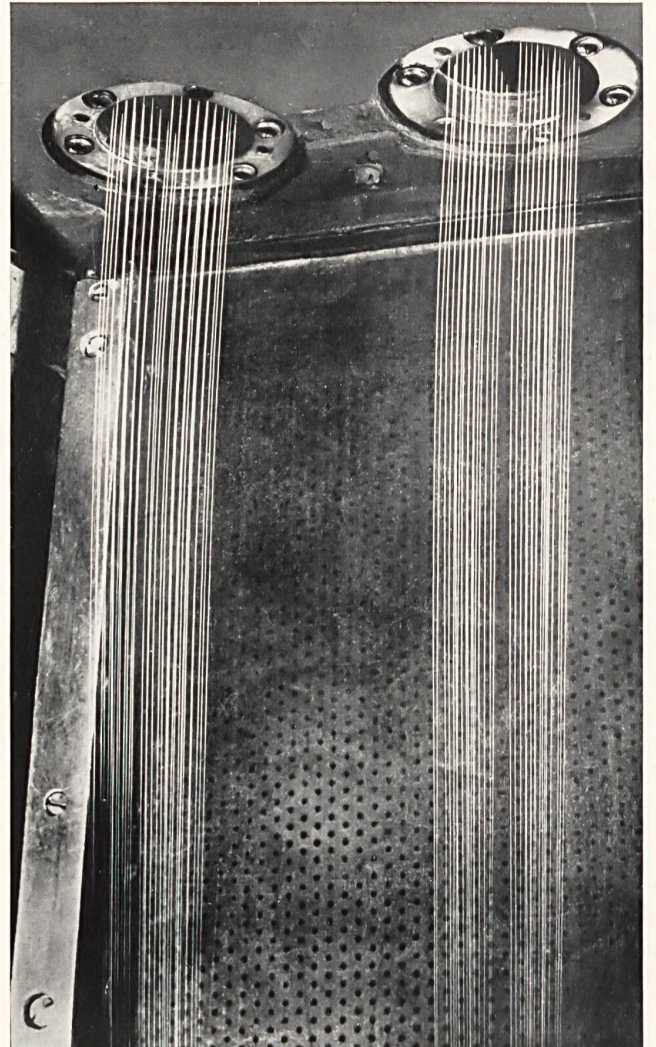
Geschmolzenes Nylon wird aus den Spinnösen herausgepresst und erstarrt sofort durch Abkühlung
