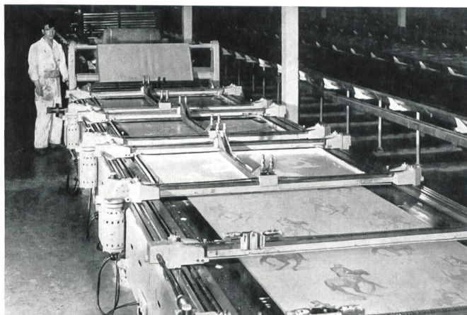
Machine moderne pour l'impression au cadre
