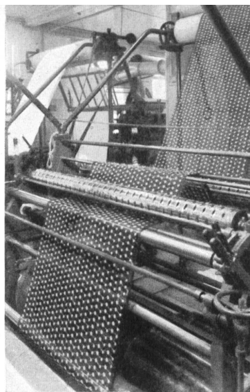
Tondeuse automatique coupant les superflus. Automatic shears cut thread ends. Una esquiladora automática corta cabos de hilo superfluos. Maschine zum Abschneiden der herau stehenden Fadendenen.
