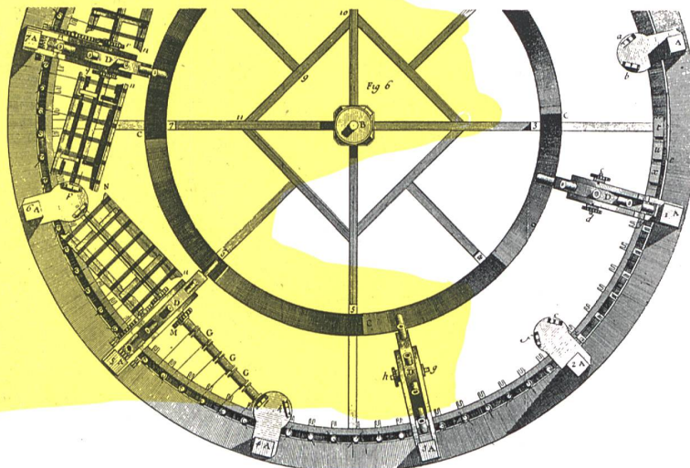
Detalle de una máquina de torcer - Grabado del siglo XVIII - Dictionnaire raisonné des sciences
