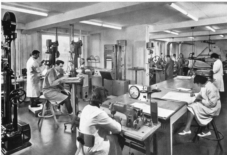
Laboratorio climatizado para el ensayo de los textiles
