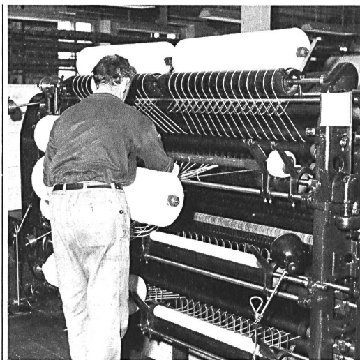
Entnahme der Vorgarne auf dem Streichgarnkrepel. Enlèvement des mèches de préparation de la cardé. Removal of the roving from the carding machine.
