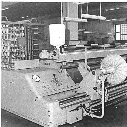
Moderne Sektionalschärmaschine zur Herstellung der Webketten. Ourdissoir sectionnel moderne pour la préparation des chaînes. Modern sectional warping frame for the production of weaving warps.
